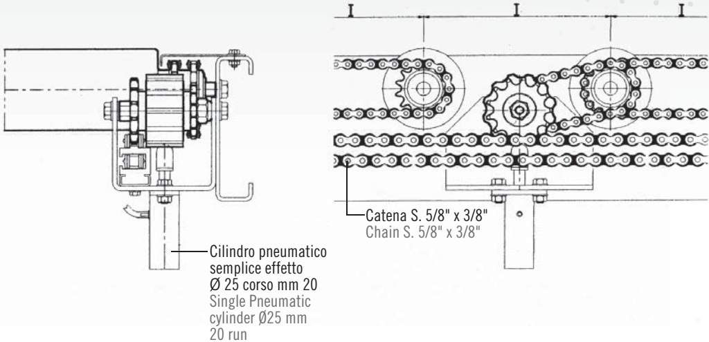
Esempi di montaggio con rulli C.I. Example of mounting with C.I. rollers
