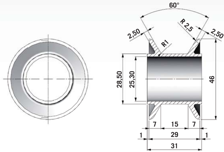
PULEGGIA IN NYLON Ø 48/25 PER RULLI FRIZIONATI CON GOLA NYLON PULLEY Ø 48/25 FOR FRICTION ROLLERS WITH GROOVES
