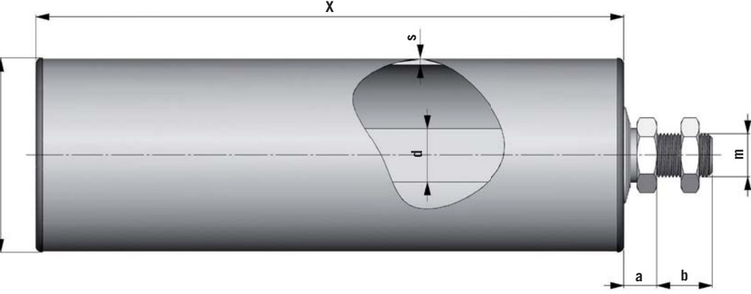
RULLO A SBALZO SIGMA - OMEGA SIGMA-OMEGA CANTILEVER ROLLER
