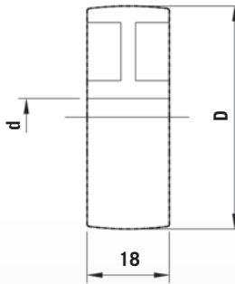
Rotelle tipo 48/8-P Type 48/8 - P skatewheel
