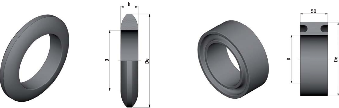
Disco tipo "B" Type B Molded disc rolls
