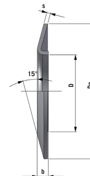
Bordini di contenimento Retaining flanges
