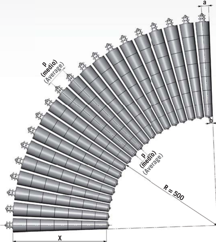
RULLI CONICI BETA CI 2R - 34 CURVA PIANA 90° TAPERED ROLLERS BETA CI 2R - 34 90° FLAT CURVE
