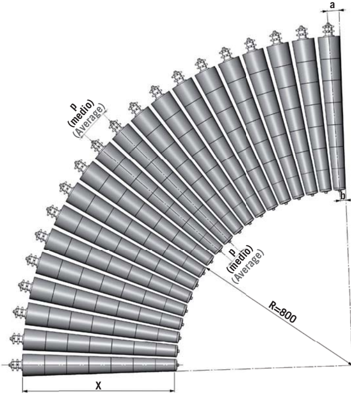
RULLI CONICI BETA3 CI 2R - 54 CURVA PIANA 90° TAPERED ROLLERS BETA 3 2R-54 90° FLAT CURVE
