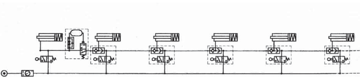
Esempi di montaggio con rulli C.E. Example of mounting with C.E. rollers
