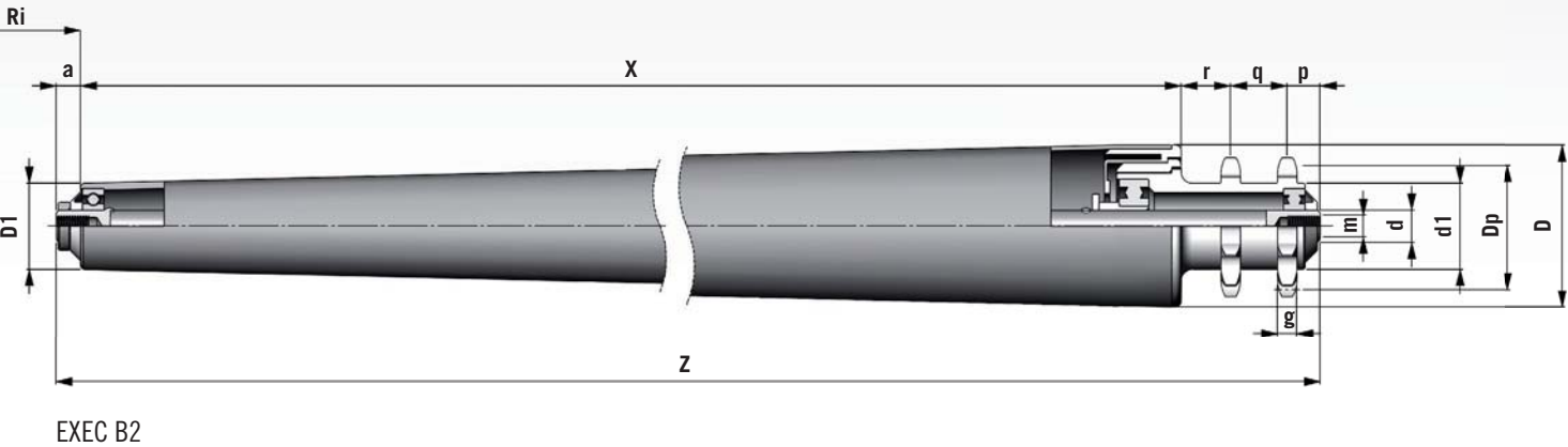
RULLO CONICO GAMMA ACCIAIO GAMMA TAPERED ROLLER
