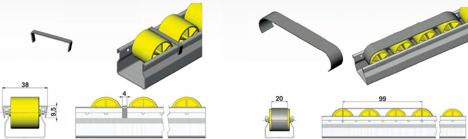
FORCELLA ANTI-APERTURA: In acciaio elastico che impedisce l'allargamento del profilo in caso di carichi eccessivi. LOCKING BRACKET: flexible steel to keep frame from expanding with heavy loads.
