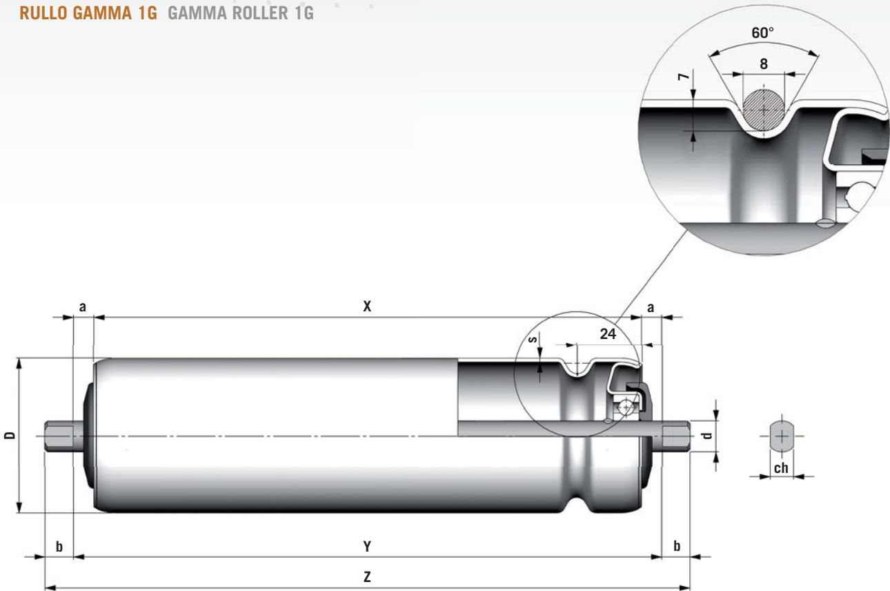
RULLO GAMMA 1G GAMMA ROLLER 1G
