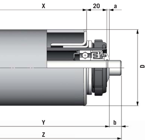
Frizione registrabile Adjustable frictioned pinion sproket
