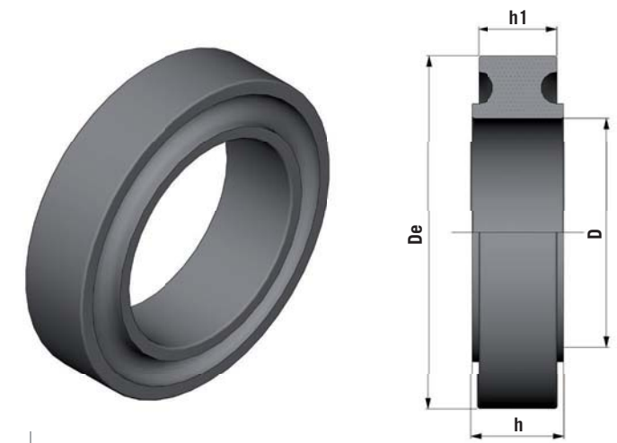
Anello d'impatto Molded roll
