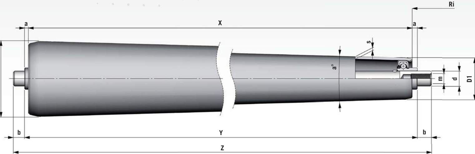
EXEC B2 ACCIAIO EXEC B2 STEEL
