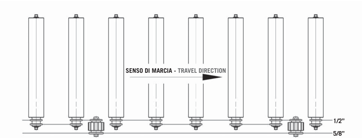
Ruote frizione destre (DX) Right friction sprockets (DX)
