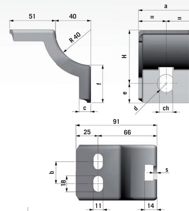
Supporto 600.3 per stazioni inferiori Support 600.3 for lower stations
