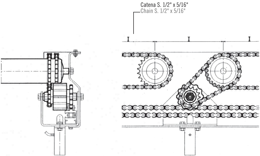
Esempi di montaggio con rulli C.I. Example of mounting with C.I. rollers
