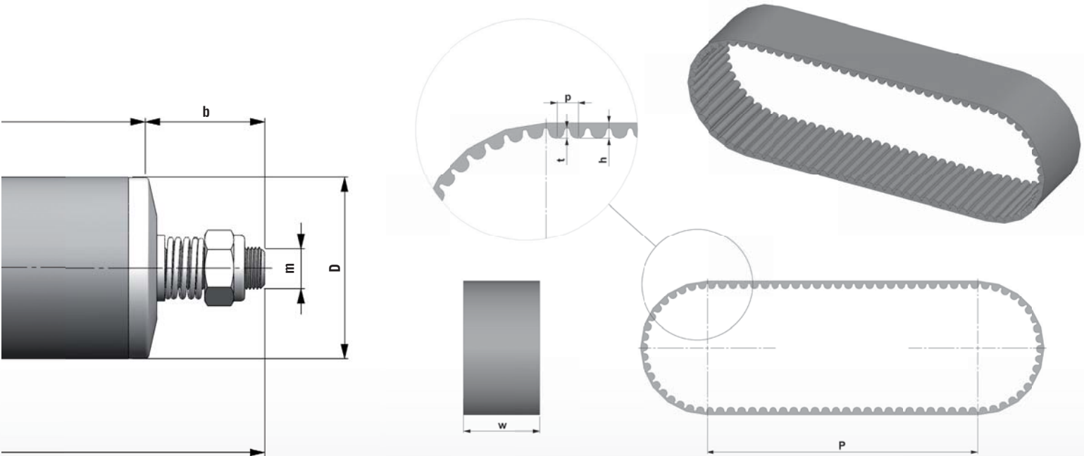
Frizione registrabile Adjustable frictioned pulley
