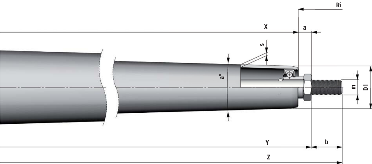
EXEC C ACCIAIO EXEC C STEEL
